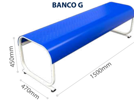
Nk 1906 BANCO G
