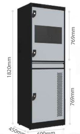
Nk 1713 RACK DE COMPUTADOR INDUSTRIAL
