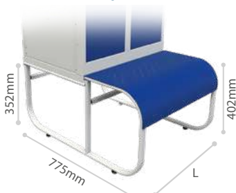
Nk 1900 ASSENTO EM AÇO GALVANIZADO
